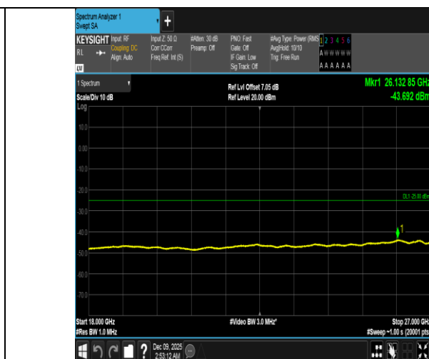
Band41-20MHz-QPSK-41490-1RB#99-18000~27000-PASS
