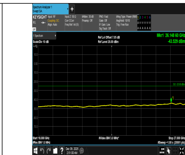
Band41-20MHz-16QAM-41490-1RB#0-18000~27000-PASS
