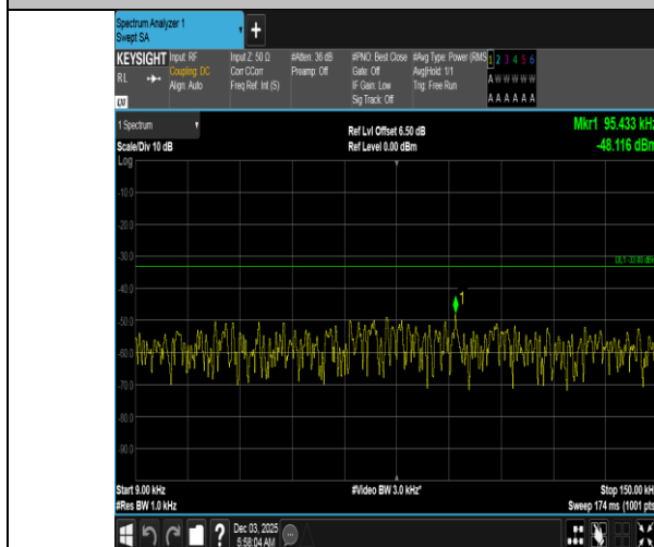
Band5-3MHz-QPSK-20635-1RB#0-0.009~0.15-PASS
