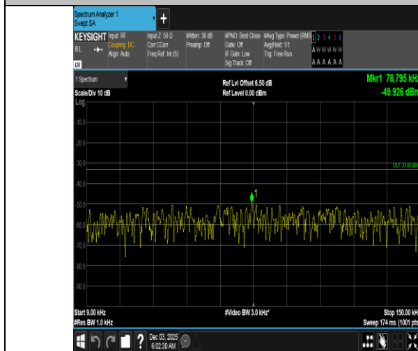
Band5-3MHz-QPSK-20635-15RB#0-0.009~0.15-PASS
