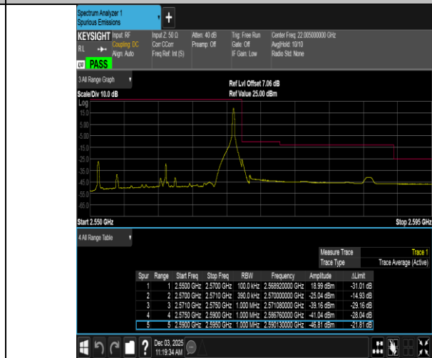
Band7-20MHz-QPSK-21350-1RB#99-PASS
