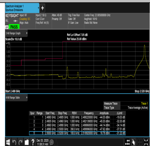
Band7-20MHz-QPSK-20850-1RB#99-PASS
