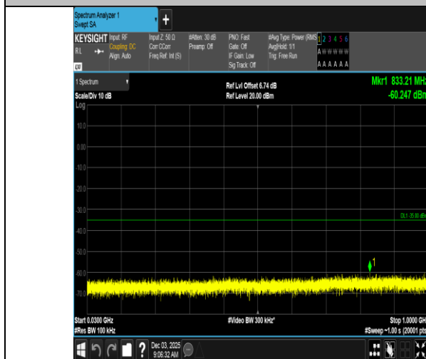
Band7-10MHz-QPSK-20800-50RB#0-30~1000-PASS
