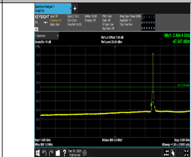
Band7-10MHz-QPSK-20800-50RB#0-1000~3000-PASS
