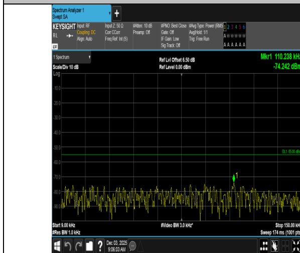
Band7-10MHz-QPSK-20800-50RB#0-0.009~0.15-PASS
