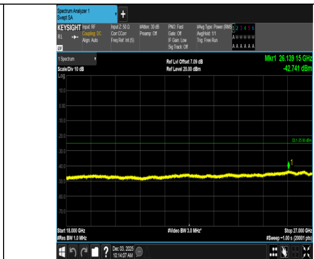
Band7-15MHz-QPSK-20825-1RB#0-18000~27000-PASS
