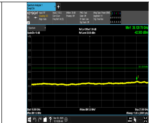
Band7-15MHz-16QAM-20825-1RB#74-18000~27000-PASS
