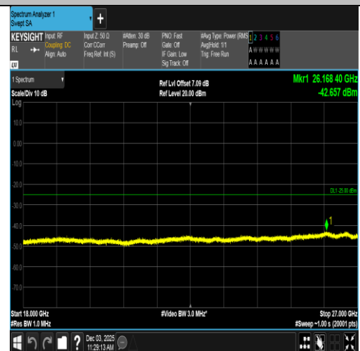
Band7-20MHz-QPSK-20850-1RB#99-18000~27000-PASS
