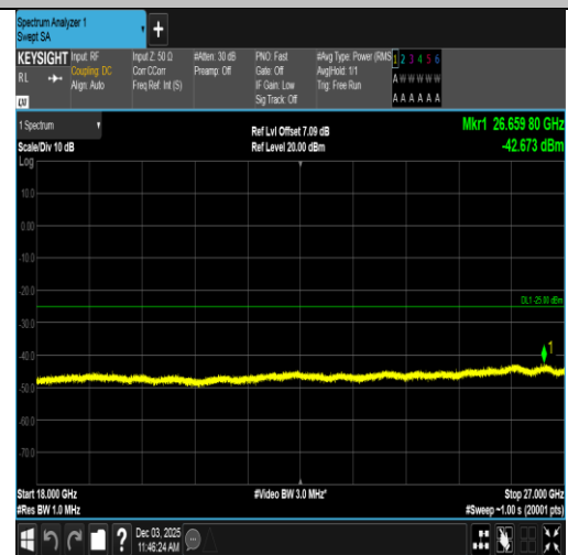
Band7-20MHz-QPSK-21350-1RB#99-18000~27000-PASS
