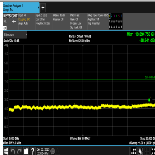
Band2-9400-3-3000~20000MHz-PASS
