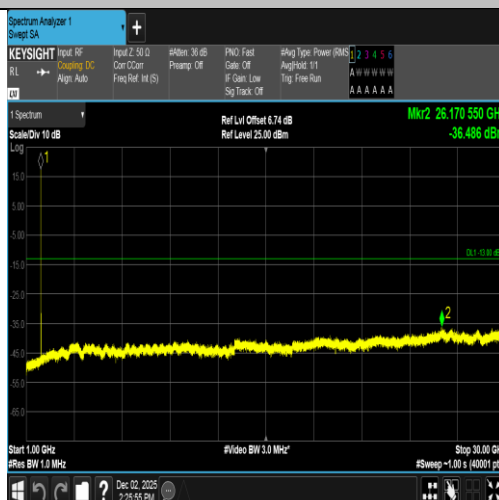
Band2-9400-1-1000~30000MHz-PASS
