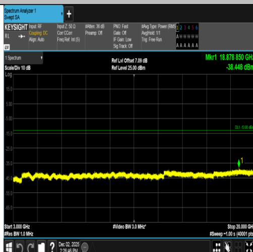
Band2-9538-1-3000~20000MHz-PASS
