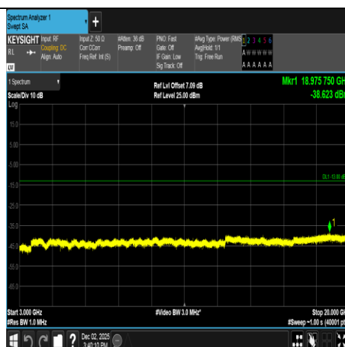
Band2-9400-3-3000~20000MHz-PASS
