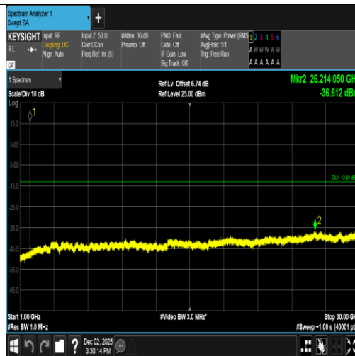
Band2-9262-1-1000~30000MHz-PASS
