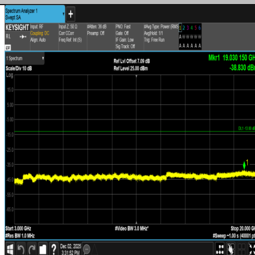
Band2-9400-1-3000~20000MHz-PASS
