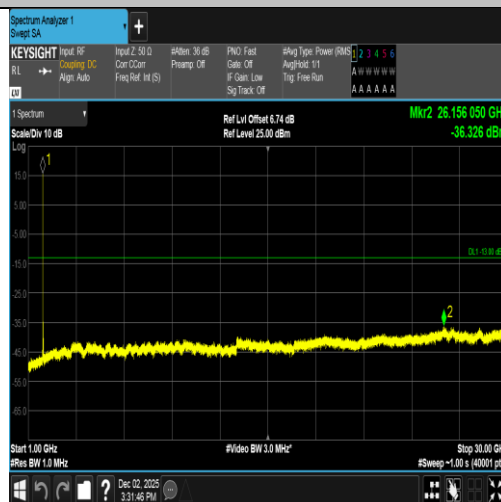
Band2-9400-1-1000~30000MHz-PASS
