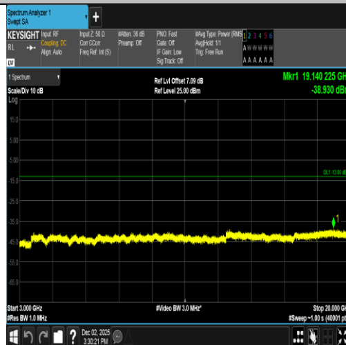
Band2-9262-1-3000~20000MHz-PASS
