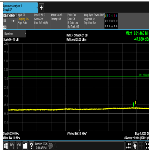
Band2-9400-1-30~1000MHz-PASS
