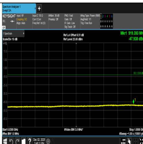
Band2-9538-5-30~1000MHz-PASS
