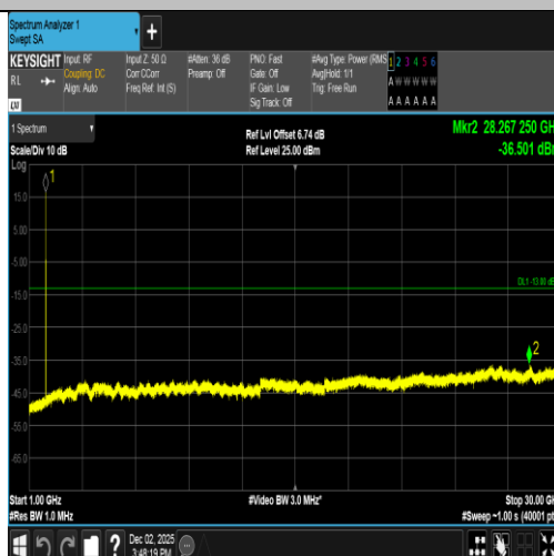
Band2-9538-5-1000~30000MHz-PASS
