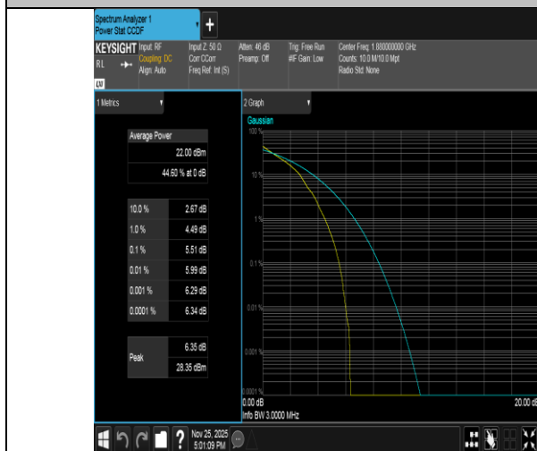
Band2-3MHz-QPSK-18900-1RB#0-PASS
