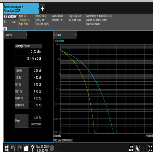
Band2-20MHz-QPSK-18700-100RB#0-PASS
