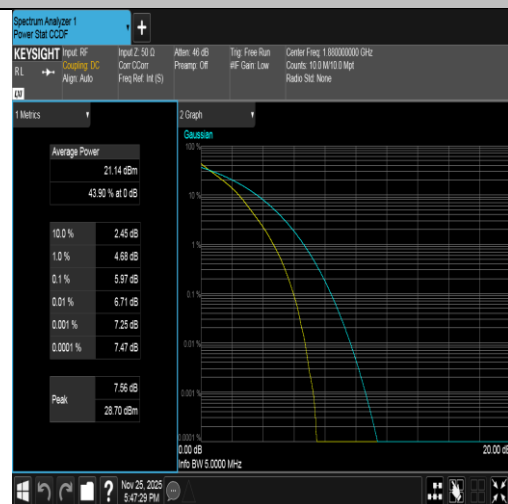
Band2-5MHz-QPSK-18900-25RB#0-PASS
