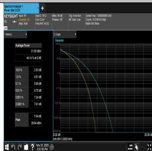
Band2-3MHz-QPSK-18900-15RB#0-PASS
