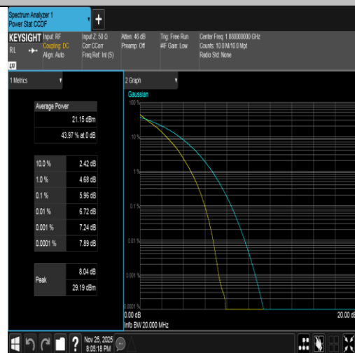
Band2-20MHz-QPSK-18900-100RB#0-PASS
