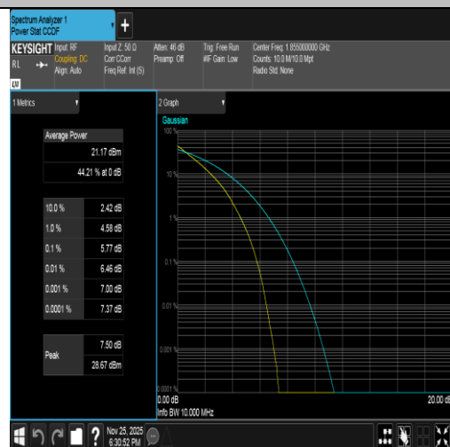
Band2-10MHz-QPSK-18650-50RB#0-PASS
