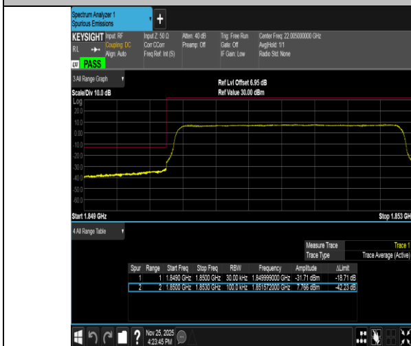
Band2-3MHz-QPSK-18615-15RB#0-PASS
