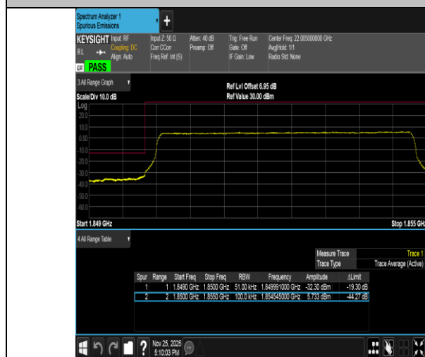
Band2-5MHz-QPSK-18625-25RB#0-PASS
