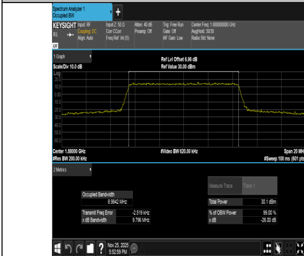
Band2-10MHz-QPSK-18900-50RB#0-PASS
