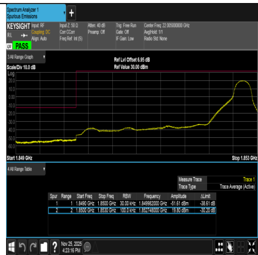
Band2-3MHz-QPSK-18615-1RB#14-PASS
