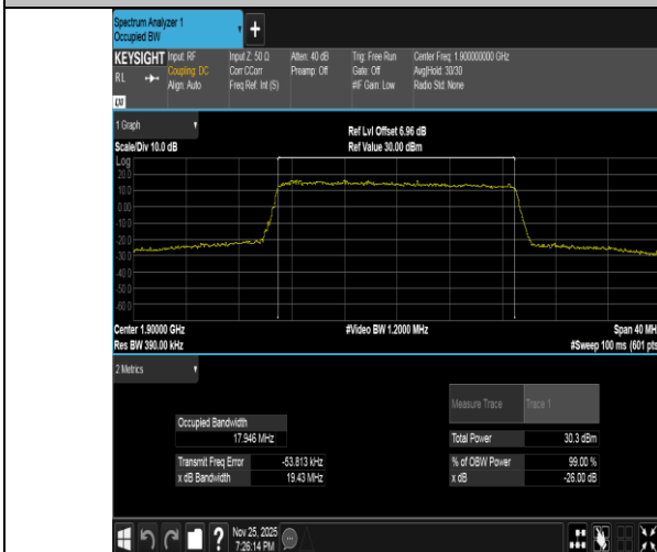
Band2-20MHz-QPSK-19100-100RB#0-PASS
