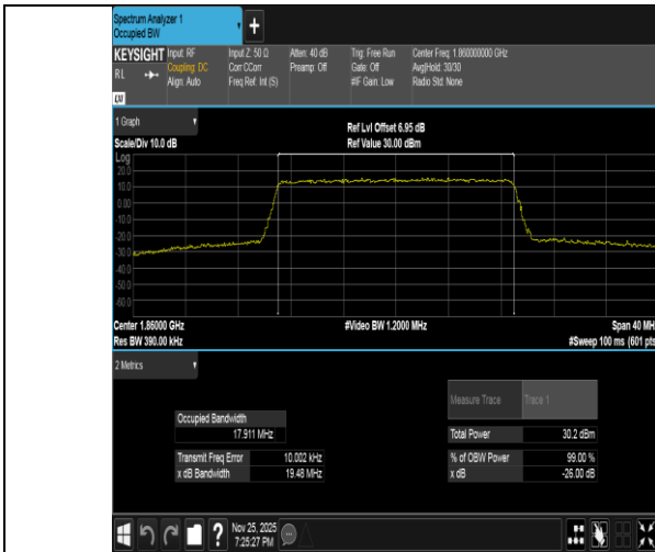
Band2-20MHz-QPSK-18700-100RB#0-PASS
