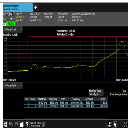
Band2-5MHz-QPSK-18625-1RB#24-PASS
