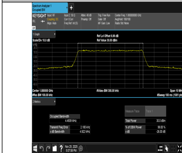
Band2-5MHz-QPSK-18900-25RB#0-PASS
