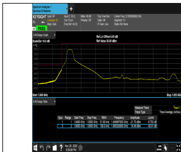
Band2-5MHz-QPSK-18625-1RB#0-PASS
