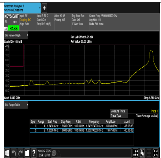
Band2-10MHz-QPSK-18650-1RB#49-PASS
