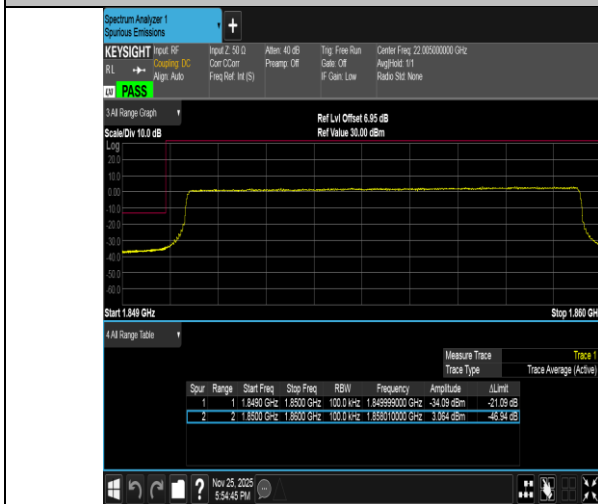
Band2-10MHz-QPSK-18650-50RB#0-PASS
