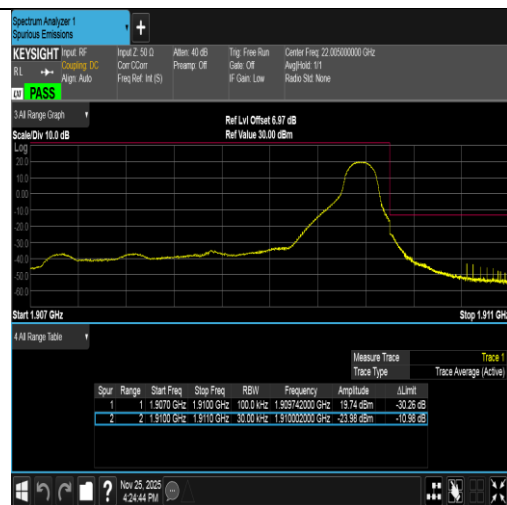
Band2-3MHz-QPSK-19185-1RB#14-PASS
