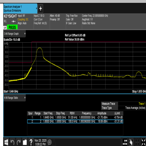
Band2-5MHz-16QAM-18625-1RB#0-PASS
