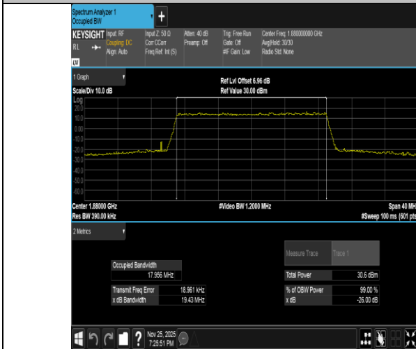
Band2-20MHz-QPSK-18900-100RB#0-PASS
