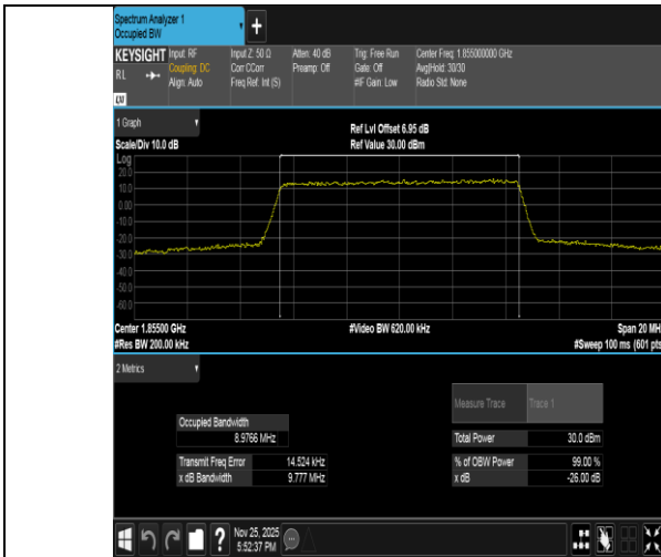
Band2-10MHz-QPSK-18650-50RB#0-PASS
