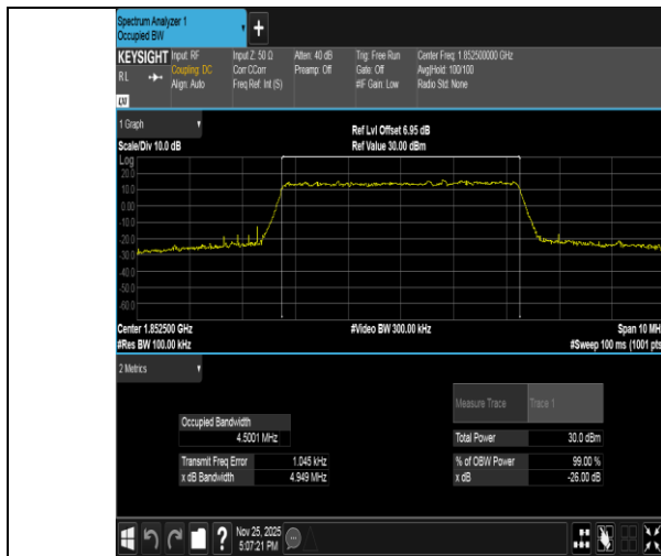
Band2-5MHz-QPSK-18625-25RB#0-PASS
