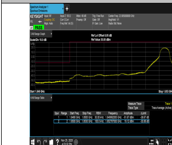
Band2-3MHz-16QAM-18615-1RB#14-PASS
