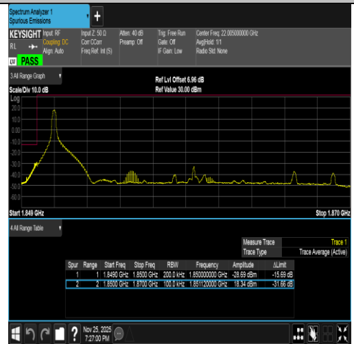
Band2-20MHz-16QAM-18700-1RB#0-PASS
