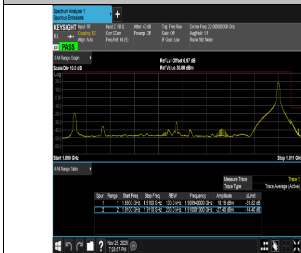
Band2-20MHz-16QAM-19100-1RB#99-PASS
