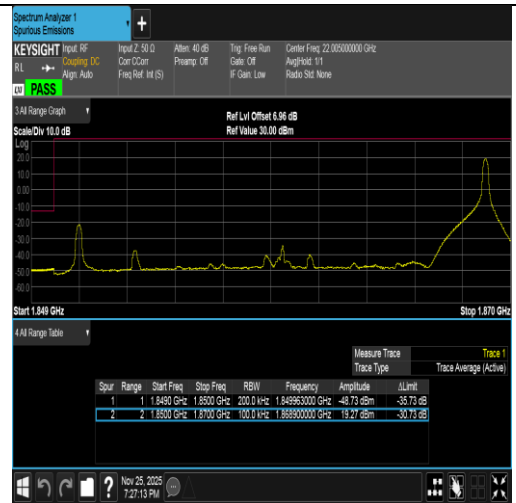
Band2-20MHz-QPSK-18700-1RB#99-PASS
