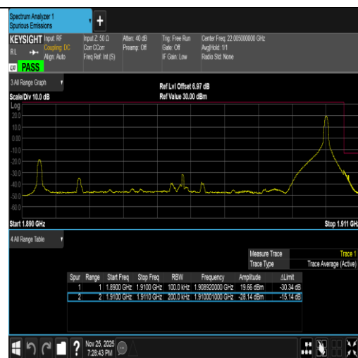
Band2-20MHz-QPSK-19100-1RB#99-PASS
