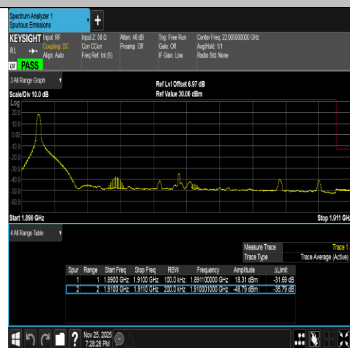
Band2-20MHz-16QAM-19100-1RB#0-PASS
