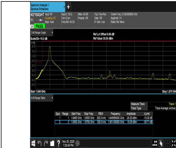
Band2-20MHz-QPSK-18700-1RB#0-PASS
