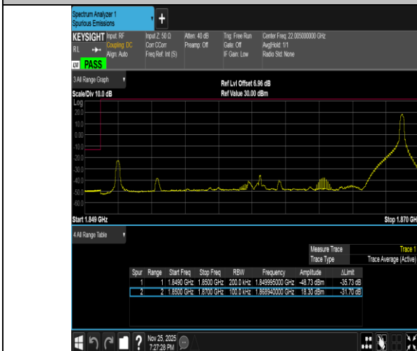
Band2-20MHz-16QAM-18700-1RB#99-PASS
