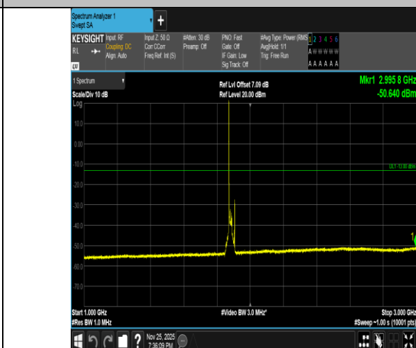
Band2-20MHz-QPSK-18900-1RB#0-1000~3000-PASS
