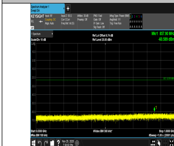
Band2-20MHz-QPSK-18700-1RB#0-30~1000-PASS
