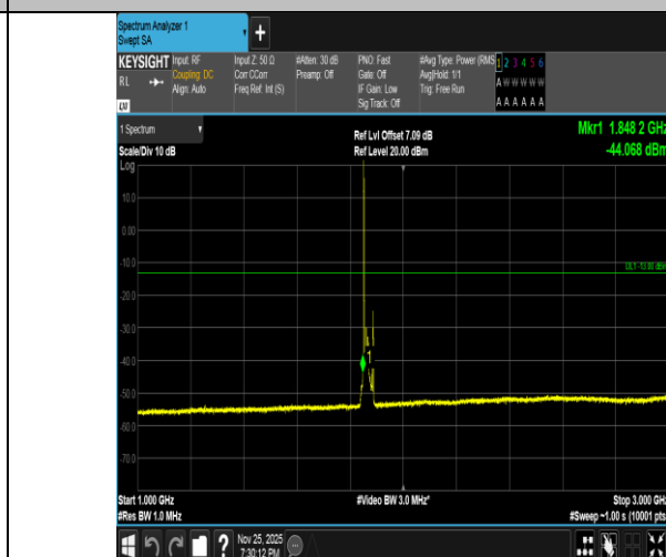
Band2-20MHz-QPSK-18700-1RB#0-1000~3000-PASS
