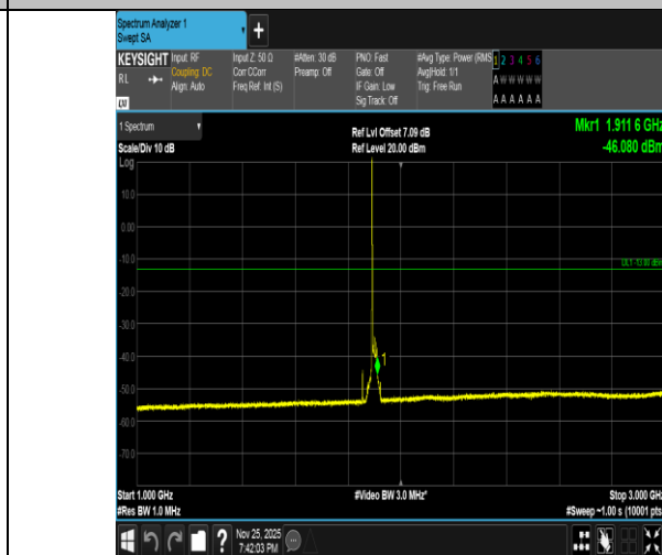
Band2-20MHz-QPSK-19100-1RB#0-1000~3000-PASS
