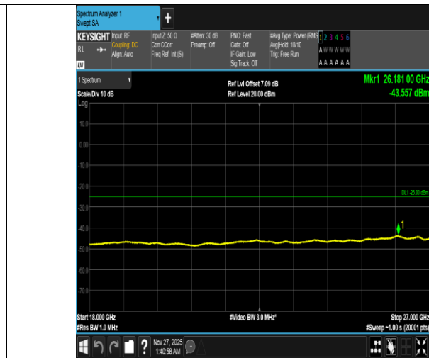
Band38-5MHz-QPSK-38000-25RB#0-18000~27000-PASS
