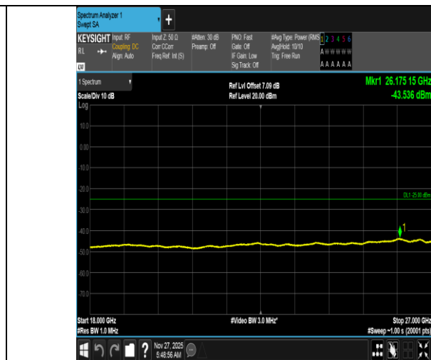
Band38-15MHz-QPSK-37825-1RB#0-18000~27000-PASS
