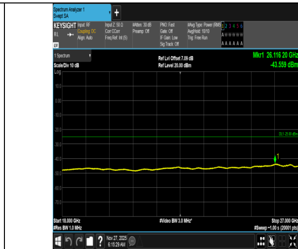
Band38-15MHz-QPSK-38000-1RB#74-18000~27000-PASS
