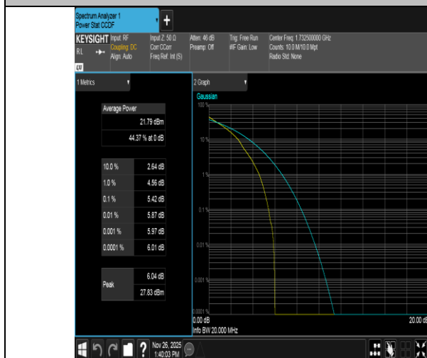
Band4-20MHz-QPSK-20175-1RB#0-PASS
