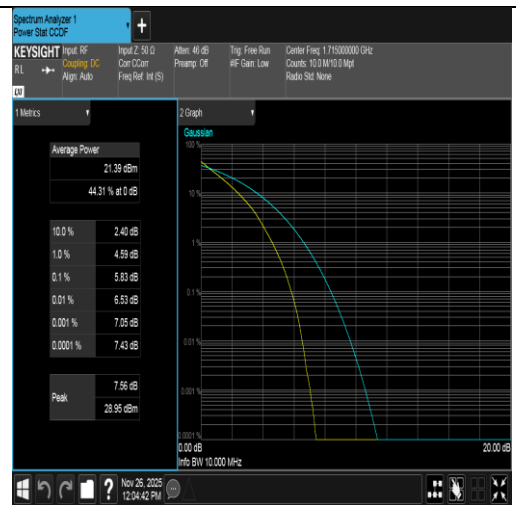
Band4-10MHz-QPSK-20000-50RB#0-PASS
