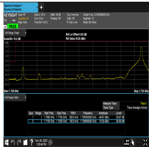
Band4-20MHz-QPSK-20050-1RB#99-PASS
