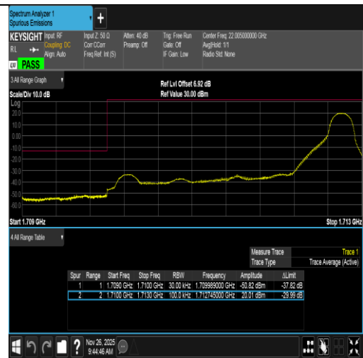
Band4-3MHz-QPSK-19965-1RB#14-PASS
