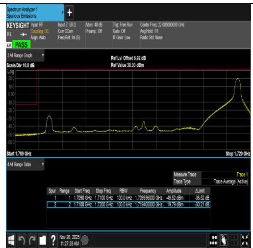
Band4-10MHz-QPSK-20000-1RB#49-PASS
