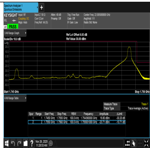
Band4-10MHz-QPSK-20350-1RB#49-PASS
