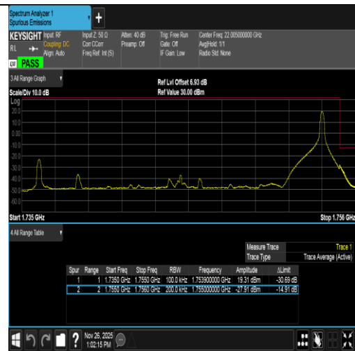
Band4-20MHz-QPSK-20300-1RB#99-PASS
