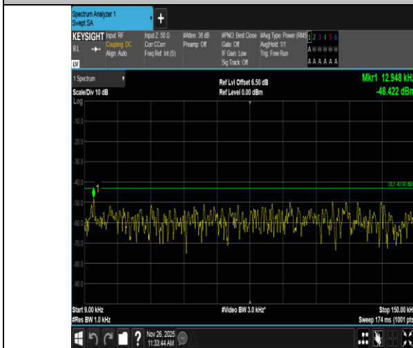
Band4-10MHz-QPSK-20000-50RB#0-0.009~0.15-PASS
