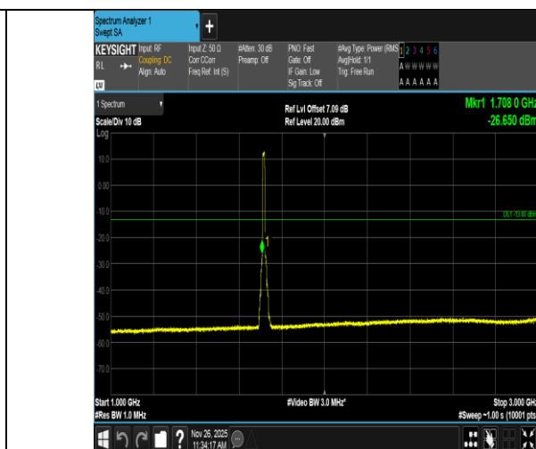
Band4-10MHz-QPSK-20000-50RB#0-1000~3000-PASS
