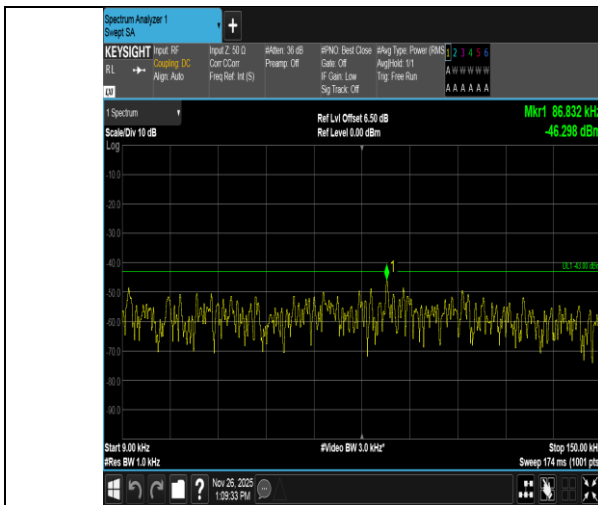
Band4-20MHz-QPSK-20175-1RB#0-0.009~0.15-PASS
