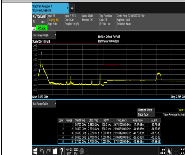
Band41-20MHz-QPSK-41490-1RB#0-PASS
