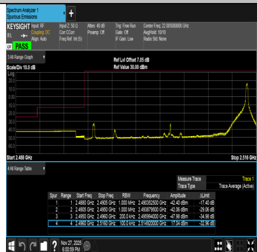
Band41-20MHz-QPSK-39750-1RB#99-PASS
