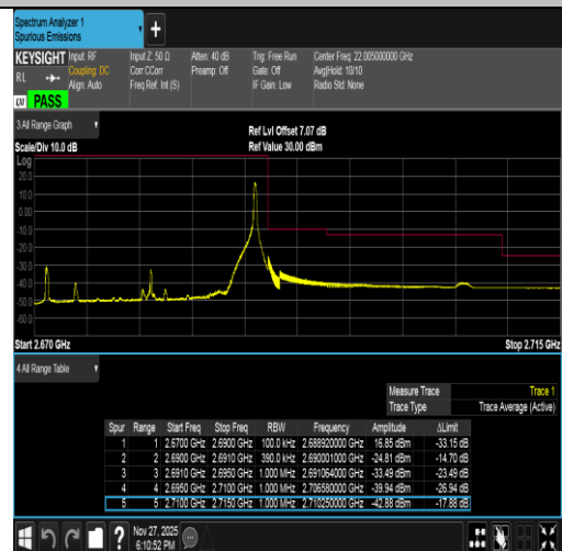
Band41-20MHz-QPSK-41490-1RB#99-PASS
