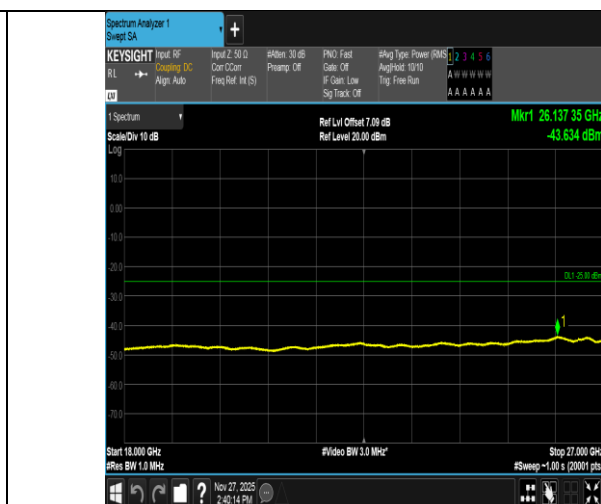
Band41-5MHz-QPSK-41565-1RB#0-18000~27000-PASS
