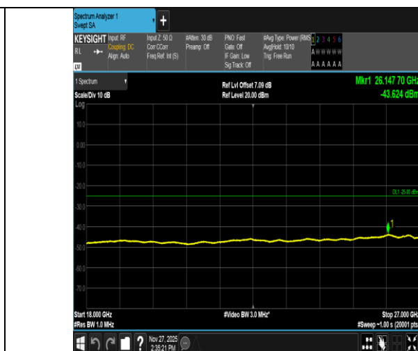
Band41-5MHz-QPSK-40620-25RB#0-18000~27000-PASS
