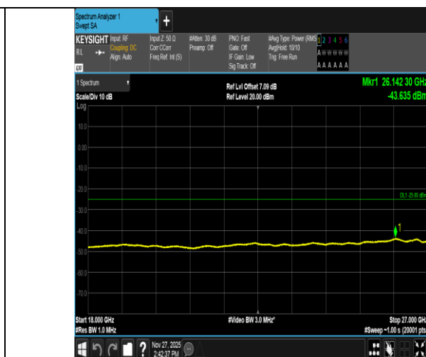
Band41-5MHz-16QAM-41565-1RB#0-18000~27000-PASS
