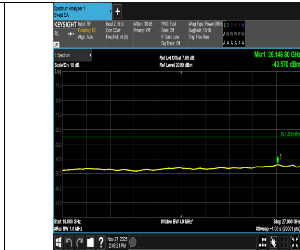
Band41-5MHz-16QAM-41565-1RB#24-18000~27000-PASS
