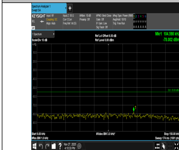
Band41-10MHz-QPSK-41540-50RB#0-0.009~0.15-PASS
