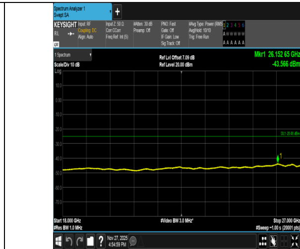
Band41-15MHz-QPSK-39725-1RB#0-18000~27000-PASS
