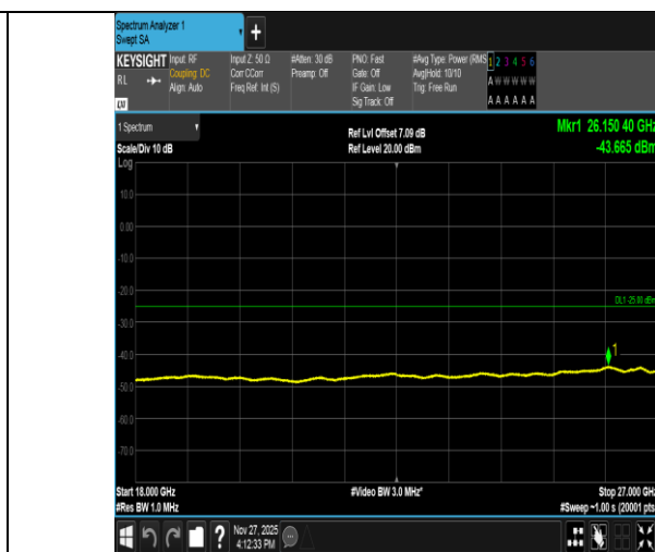
Band41-10MHz-QPSK-41540-50RB#0-18000~27000-PASS
