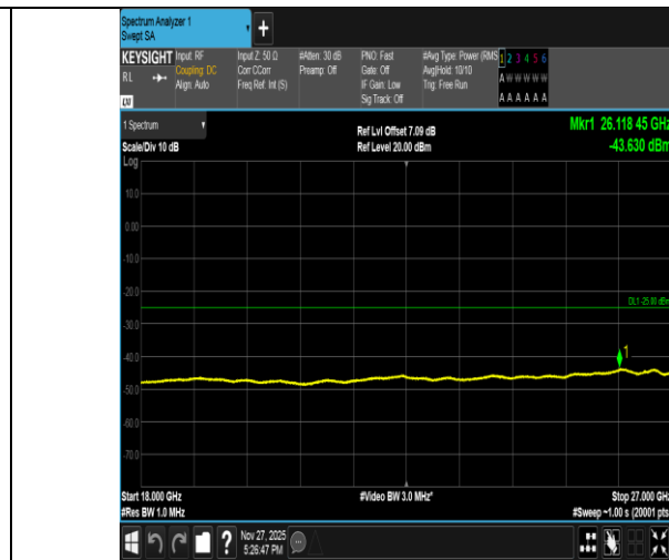
Band41-15MHz-16QAM-41515-1RB#0-18000~27000-PASS
