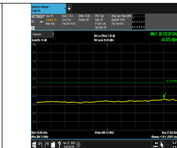
Band41-20MHz-QPSK-41490-1RB#0-18000~27000-PASS
