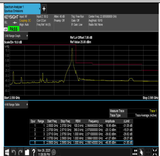
Band7-20MHz-QPSK-21350-1RB#99-PASS
