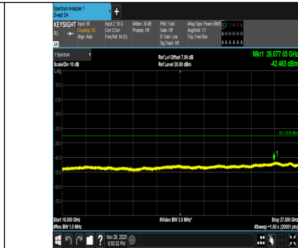
Band7-10MHz-QPSK-20800-50RB#0-18000~27000-PASS
