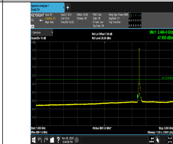
Band7-10MHz-QPSK-20800-50RB#0-1000~3000-PASS
