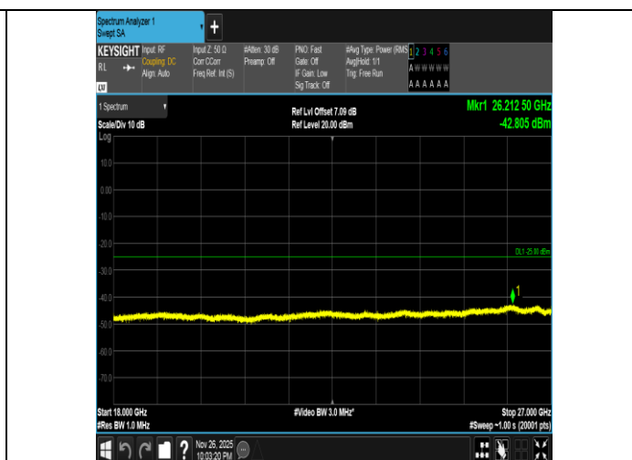
Band7-15MHz-16QAM-20825-1RB#74-18000~27000-PASS
