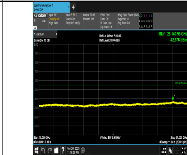
Band7-20MHz-QPSK-20850-1RB#99-18000~27000-PASS
