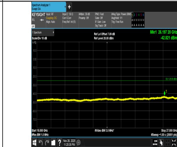
Band7-20MHz-QPSK-21100-1RB#99-18000~27000-PASS
