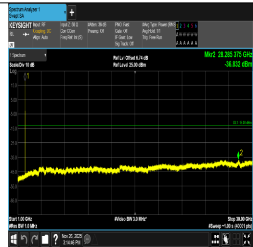
Band2-9538-1000~30000MHz-PASS
