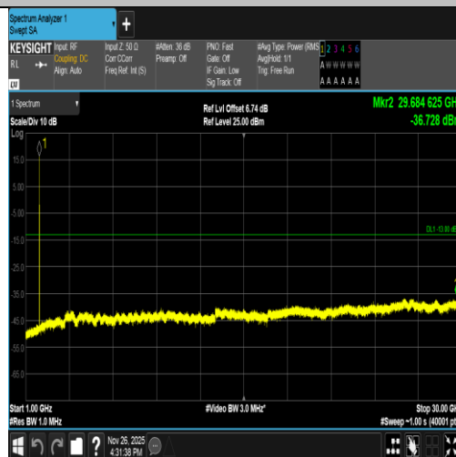
Band2-9538-4-1000~30000MHz-PASS
