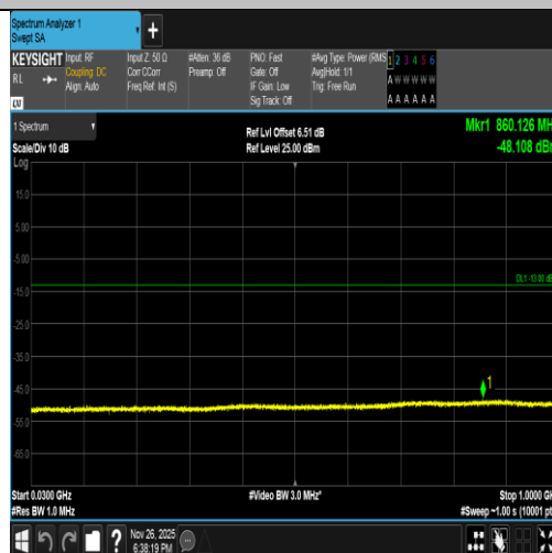
Band2-9538-3-30~1000MHz-PASS
