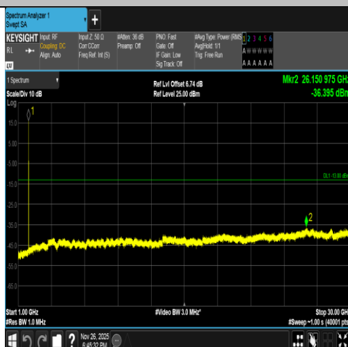
Band2-9538-5-1000~30000MHz-PASS
