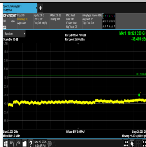
Band2-9538-2-3000~20000MHz-PASS
