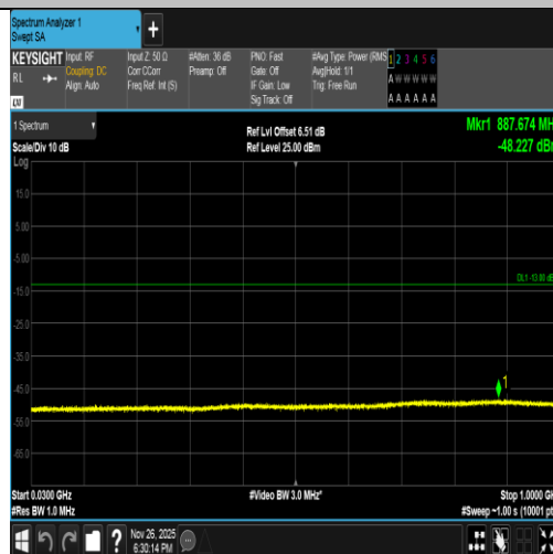
Band2-9538-1-30~1000MHz-PASS
