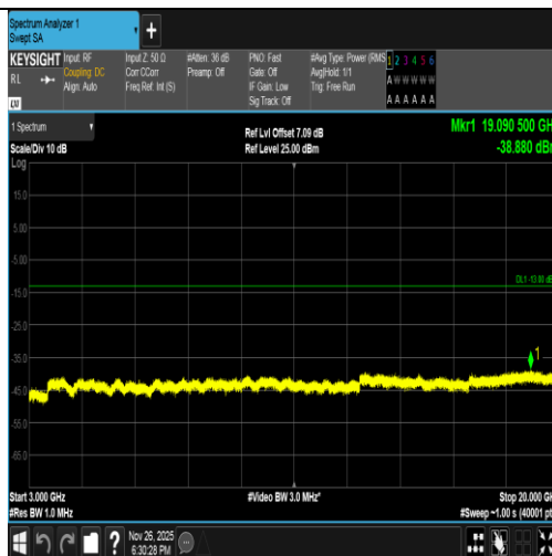
Band2-9538-1-3000~20000MHz-PASS
