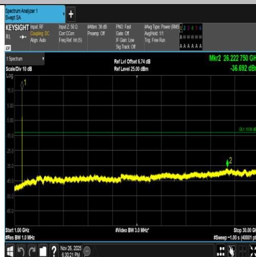
Band2-9538-1-1000~30000MHz-PASS
