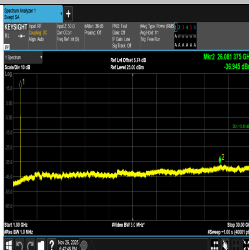
Band2-9538-4-1000~30000MHz-PASS
