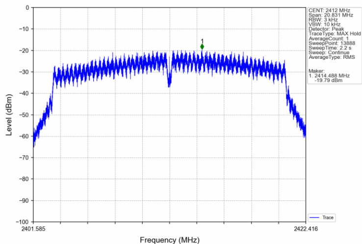
802.11n(HT20)_LCH_2412MHz_Ant2 (MIMO)_NTNV
