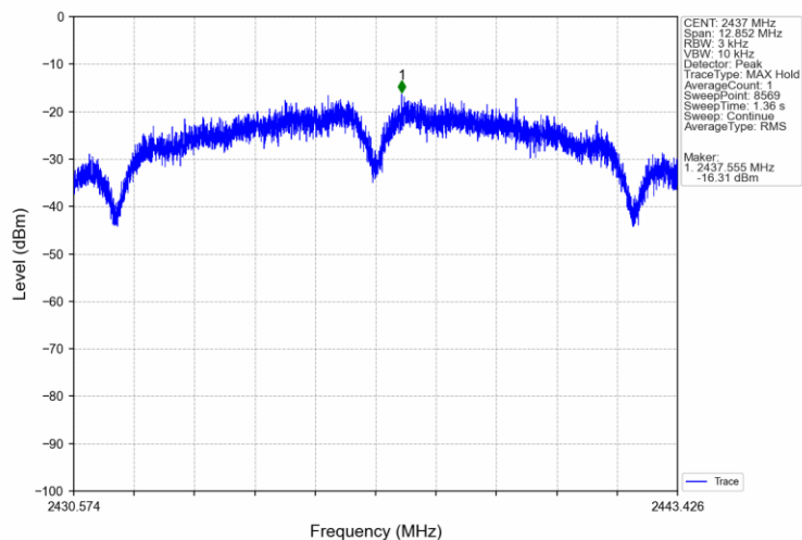
802.11g_MCH_2437MHz_Ant2 (SISO)_NTNV
