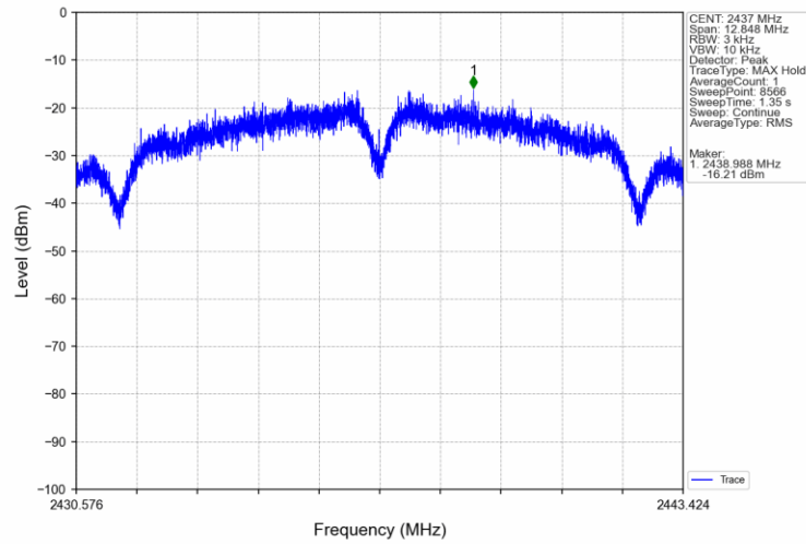
802.11b_MCH_2437MHz_Ant2 (SISO)_NTNV
