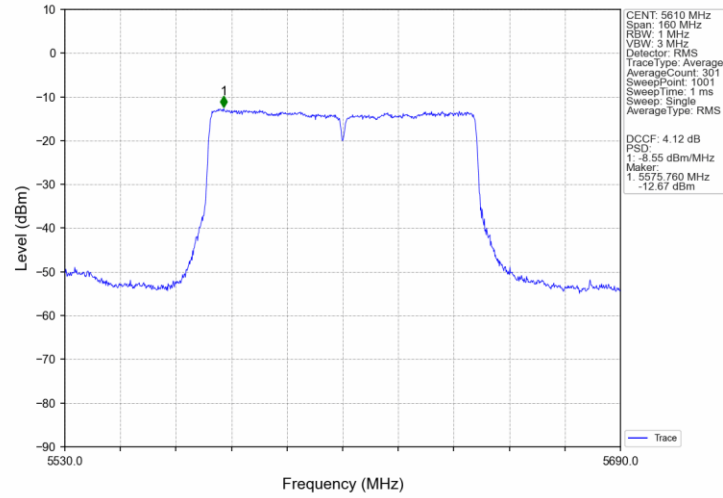
802.11ac(VHT80)_HCH_5610MHz_MIMO_NTNV
