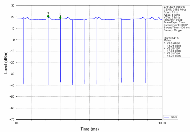
802.11b HCH 2462MHz Ant1 (SISO) NTN
