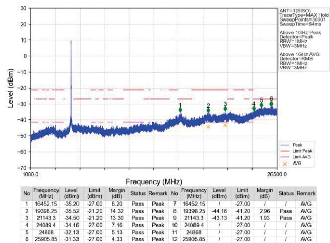
802.11a_MCH_5200MHz_Ant1_NTNV
