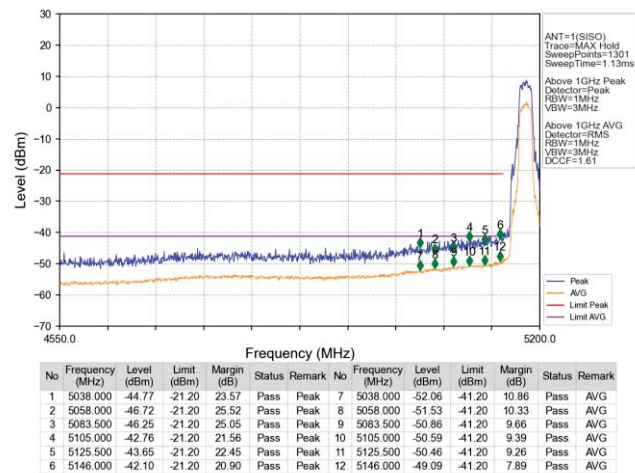
802.11a_MCH_5200MHz_Ant1_NTNV
