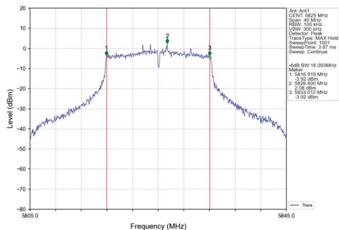
802.11a HCH_5825MHz_Ant1_NTNV
