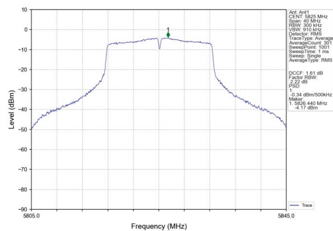
802.11a HCH_5825MHz_Ant1_NTNV
