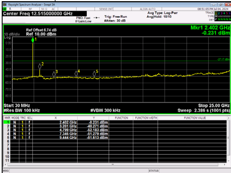
Tx. Spurious NVNT BLE 2402MHz Ant1 Emission
