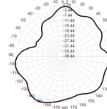
880.0MHz Total(E2-YZ), Max= 0.56dB
