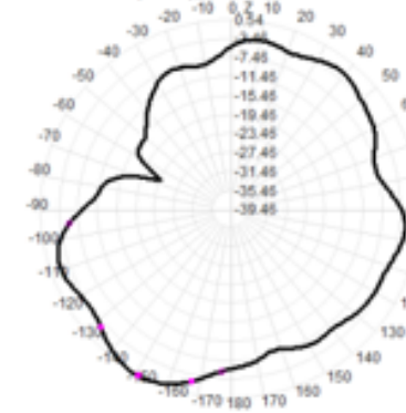
960.0MHz Total(E2-YZ), Max= 0.54dB
