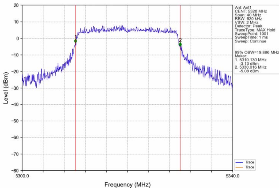
802.11ax(HEW20)_HCH_5320MHz_RU242_Left_Ant1_NTNV
