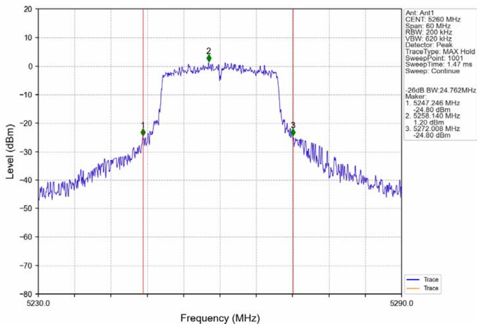
802.11ax(HEW20)_LCH_5260MHz_RU242_Left_Ant1_NTNV
