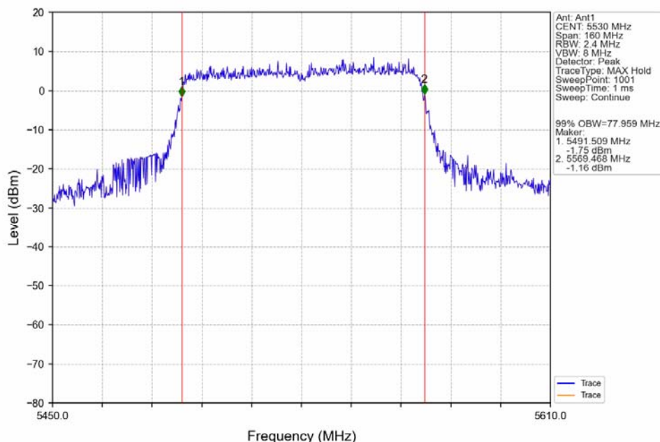
802.11ac(VHT80)_LCH_5530MHz_Ant1_NTNV
