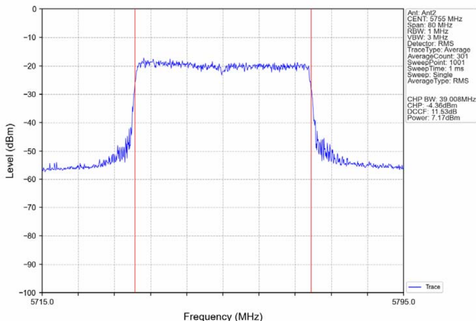
802.11ax(HEW40)_LCH_5755MHz_RU484_Left_Ant2_NTNV
