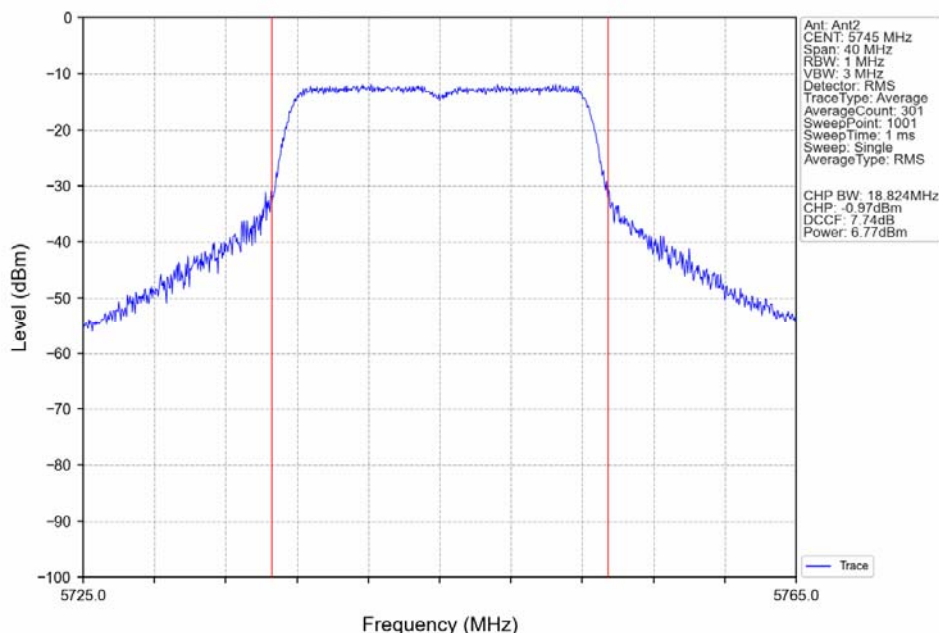
802.11a_LCH_5745MHz_Ant2_NTNV
