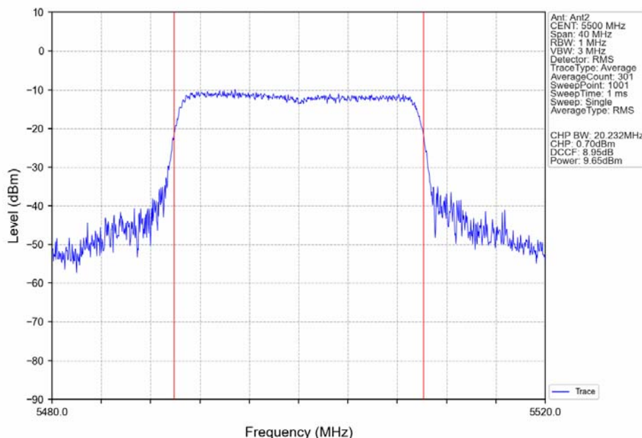
802.11ax(HEW20)_LCH_5500MHz_RU242_Left_Ant2_NTNV
