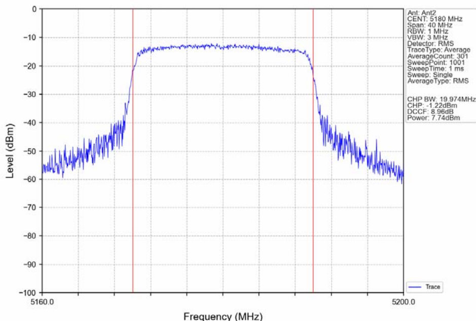
802.11ax(HEW20)_LCH_5180MHz_RU242_Left_Ant2_NTNV
