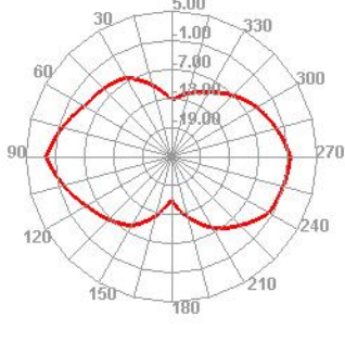
5850.000MHz H
