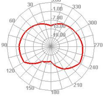
5500.000MHz E2
