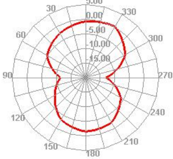
5150.000MHz E1
