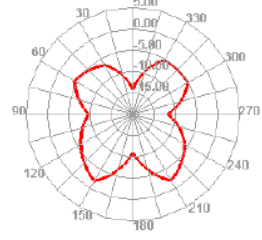
2450.000MHz E2
