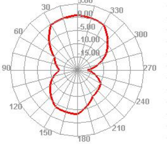
5850.000MHz E1
