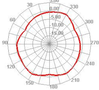
5150.000MHz E2
