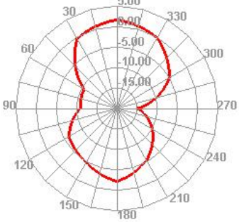
5500.000MHz E1
