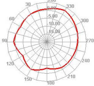
5850.000MHz E2
