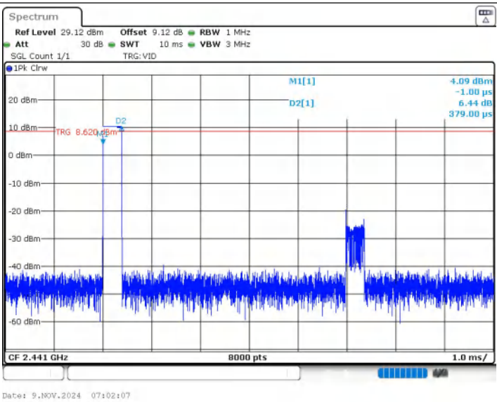
DH1_Ant1_Hop
