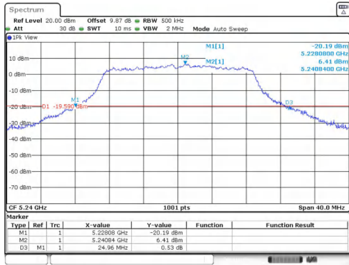
11AC20MIMO_Ant1_5240
