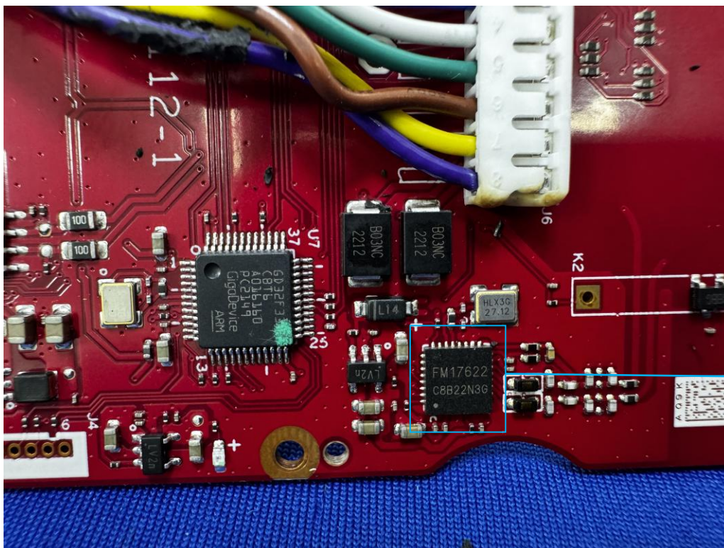
6) EUT Photo
