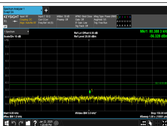
EGPRS1900-810-2-0.009~0.15MHz-PASS
