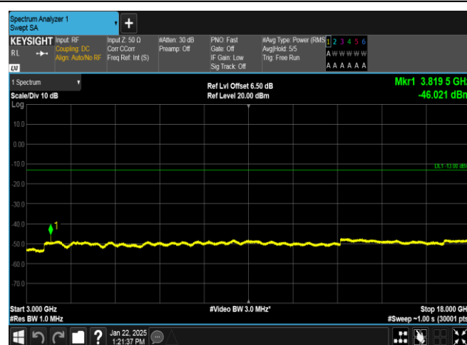
EGPRS1900-810-2-3000~18000MHz-PASS
