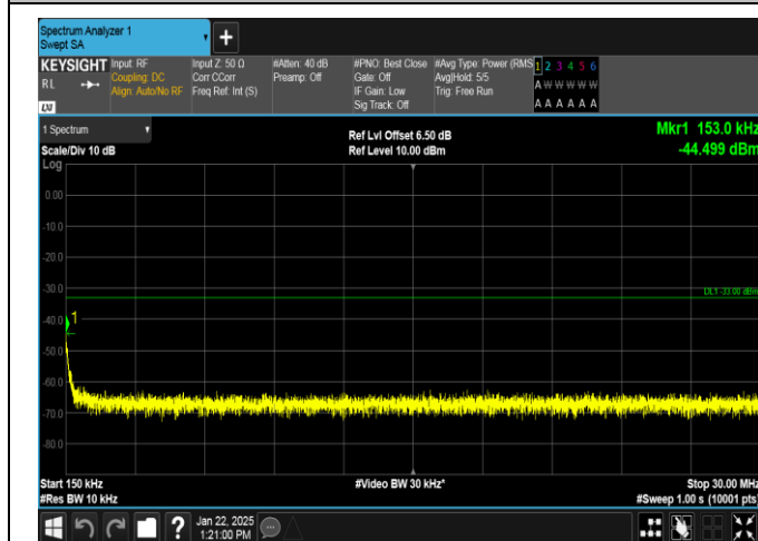
EGPRS1900-810-2-0.15~30MHz-PASS
