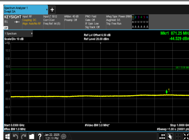
EGPRS1900-810-2-30~1000MHz-PASS
