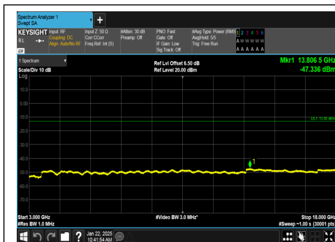
GPRS1900-810-0-3000~18000MHz-PASS
