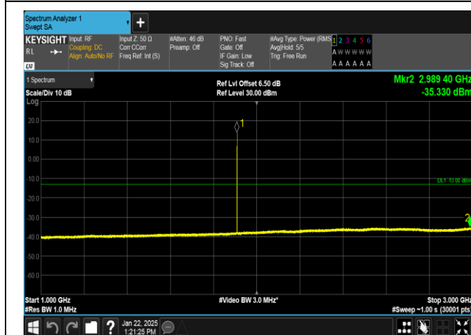
EGPRS1900-810-2-1000~3000MHz-PASS
