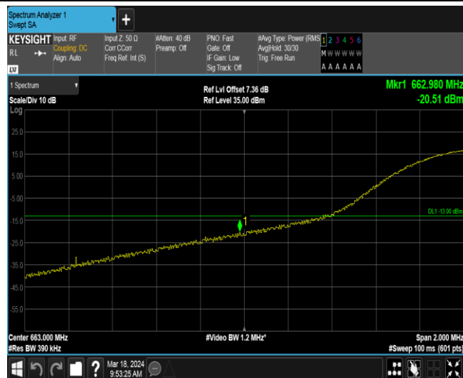
Band71-20MHz-QPSK-133222-1RB#99
