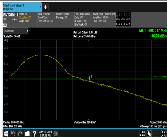
Band71-10MHz-QPSK-133422-50RB#0
