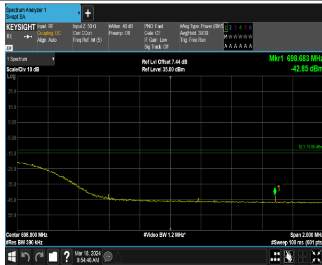
Band71-20MHz-16QAM-133372-1RB#99
