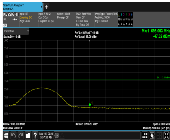
Band71-10MHz-QPSK-133422-1RB#49
