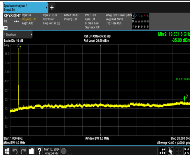
Band2-9538-1-1000~20000MHz
